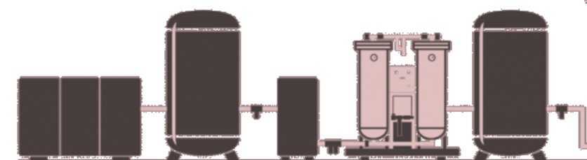
Kompresor Vzdušník Sušička Generátor Zásobník dusíku
